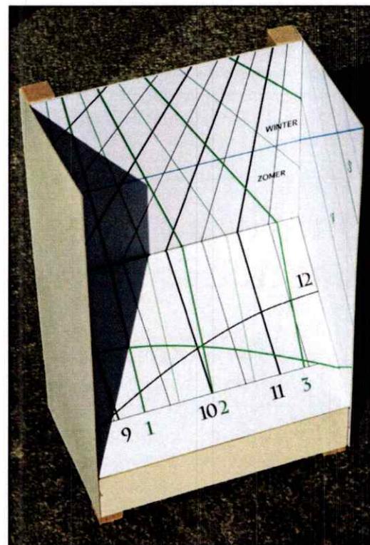
Foto van zonnwijzer-maquette nr. 82 (om 14.00 h stipt). Afmetingen (h x b): - middenvlak: 15 x 18,6 cm. - dwarsvlakken: 15, resp. 25 x 10 cm. - hellend vlak ( 45^\circ ): 10 x 18,8 cm (ware grootte: 14,14 x 18,8 cm). - totale hoogte: 30 cm.
