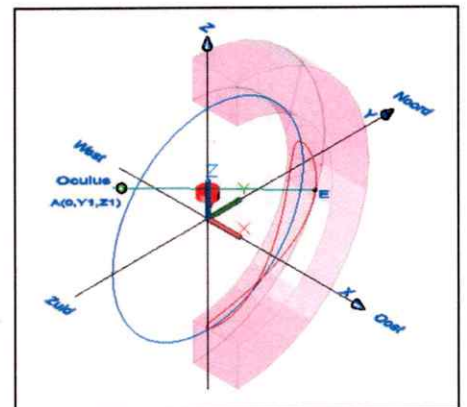
3 - Computersimulatie analemma met middaglijn op binnenzijde van halve ring (oculus vervangen door kogeltje).
