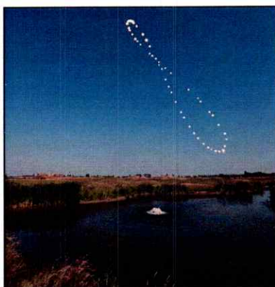
1 - Analemma van de zon om 9:00:00 (UTC) op bepaalde tijdstippen in de loop van het jaar.
